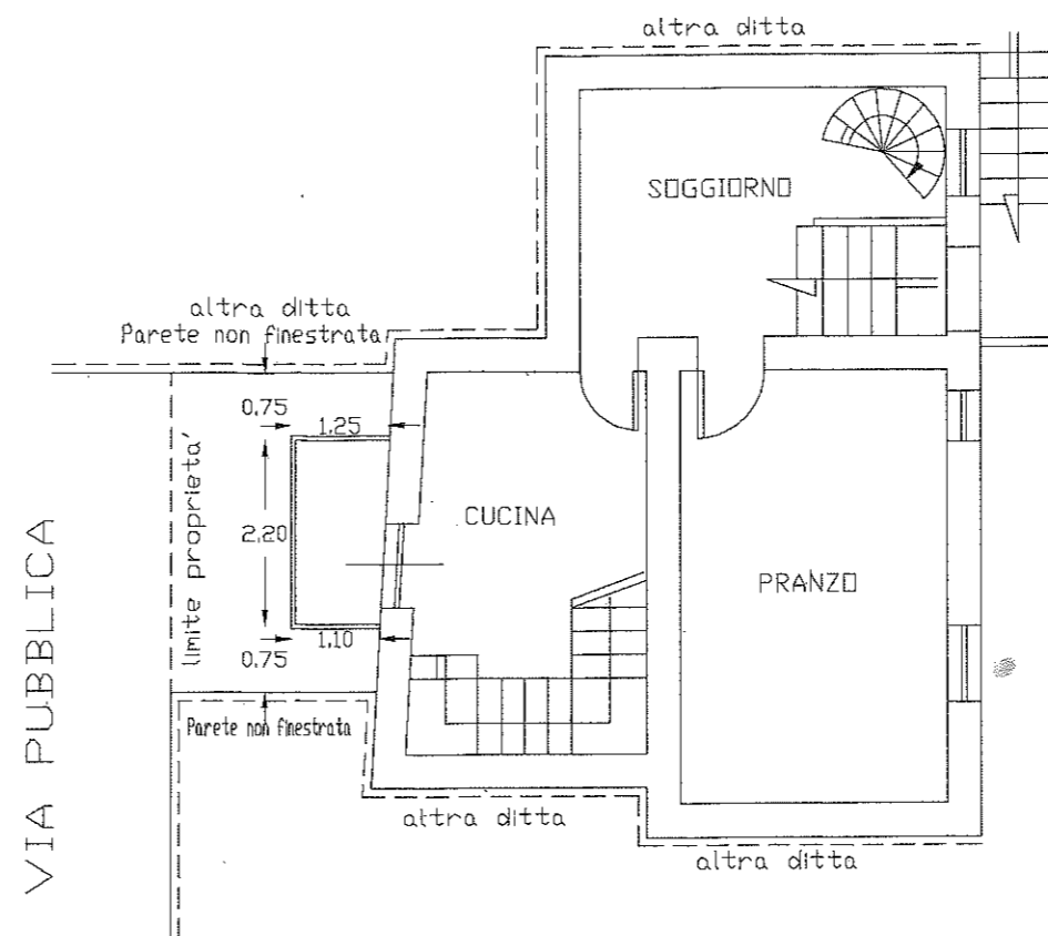
PIANO TERRA-RIALZATO
