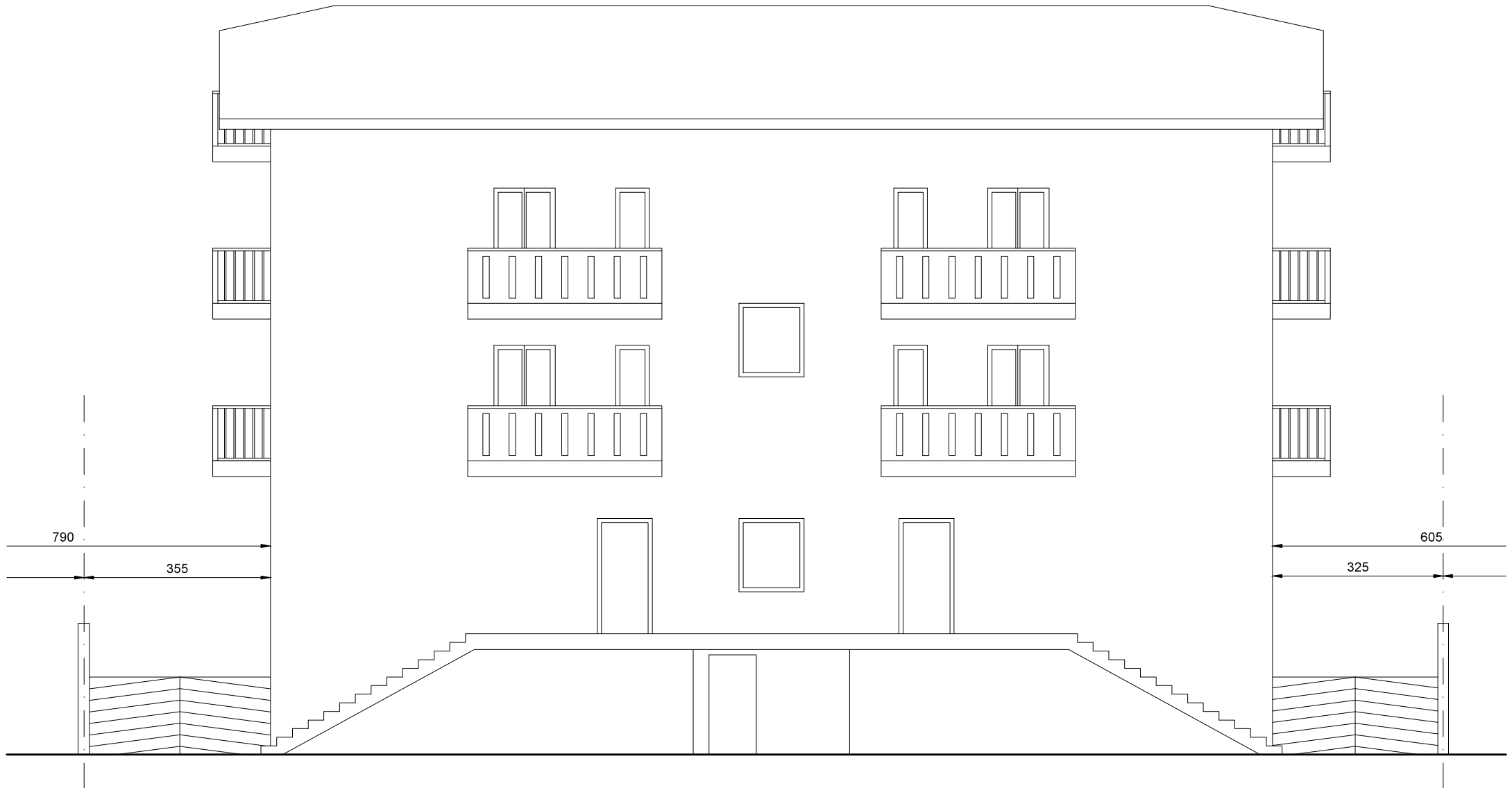
PROSPETTO NORD
