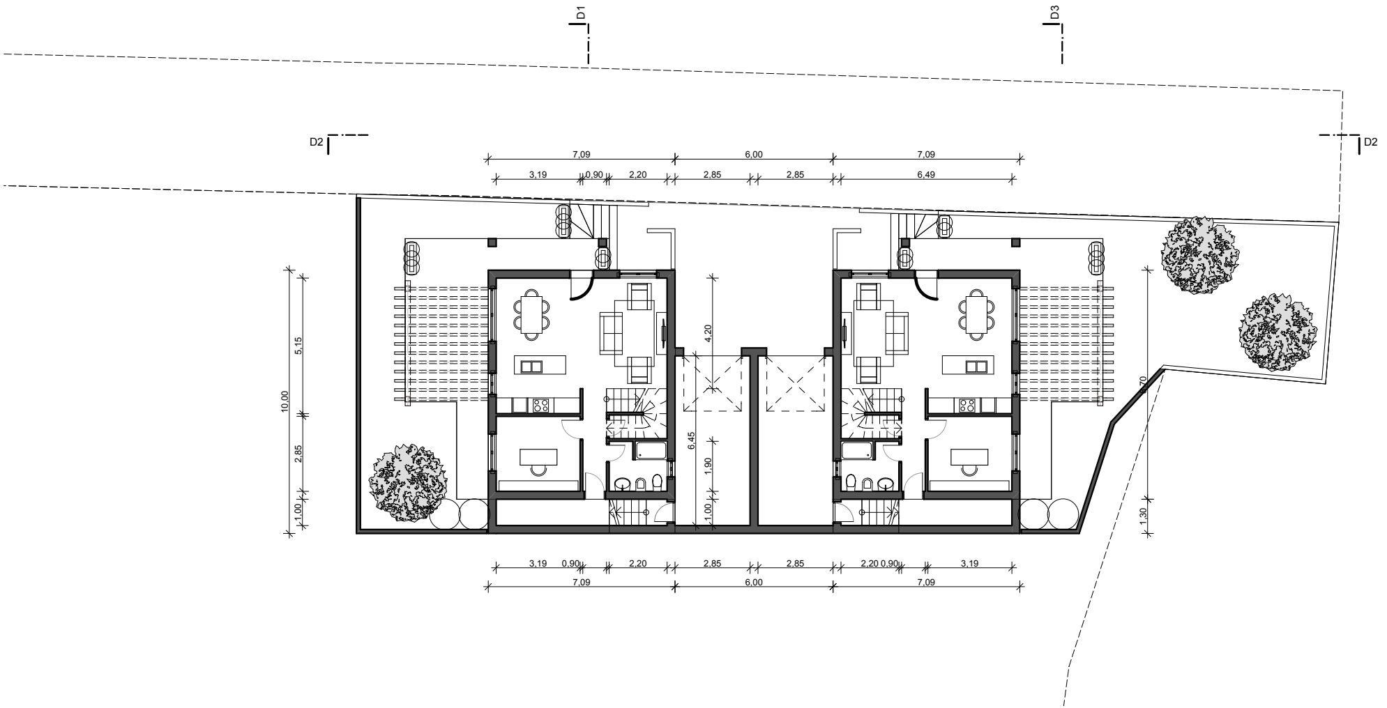
PLANIMETRIA (sistemazione esterna) - scala 1:200
